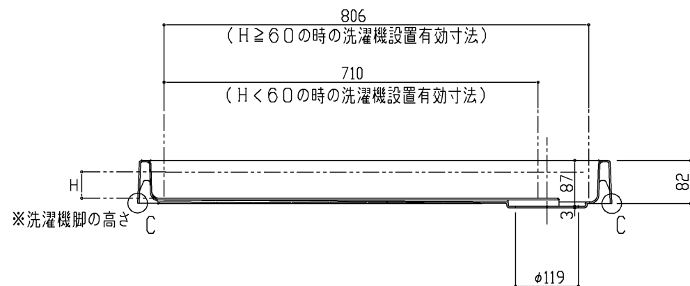
断面A-A
